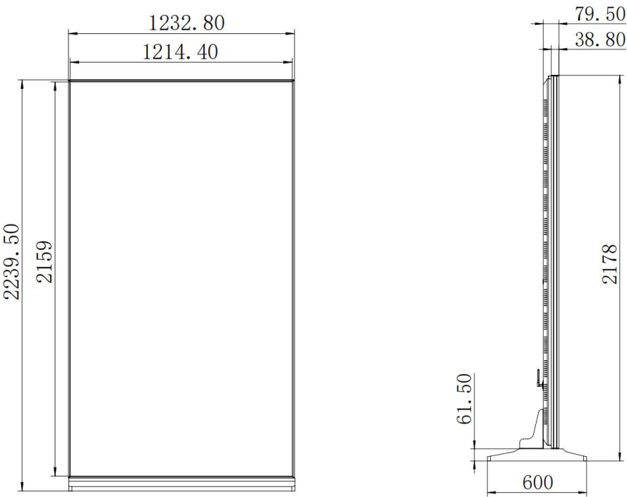
98英寸外观尺寸图
