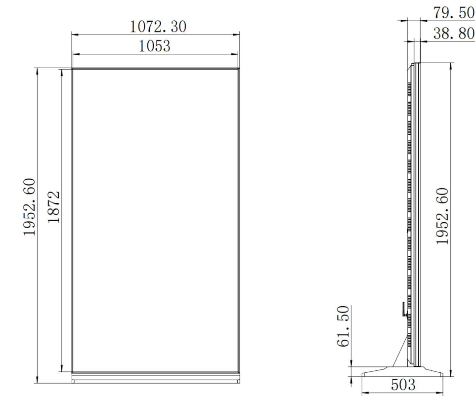
85英寸外观尺寸图
