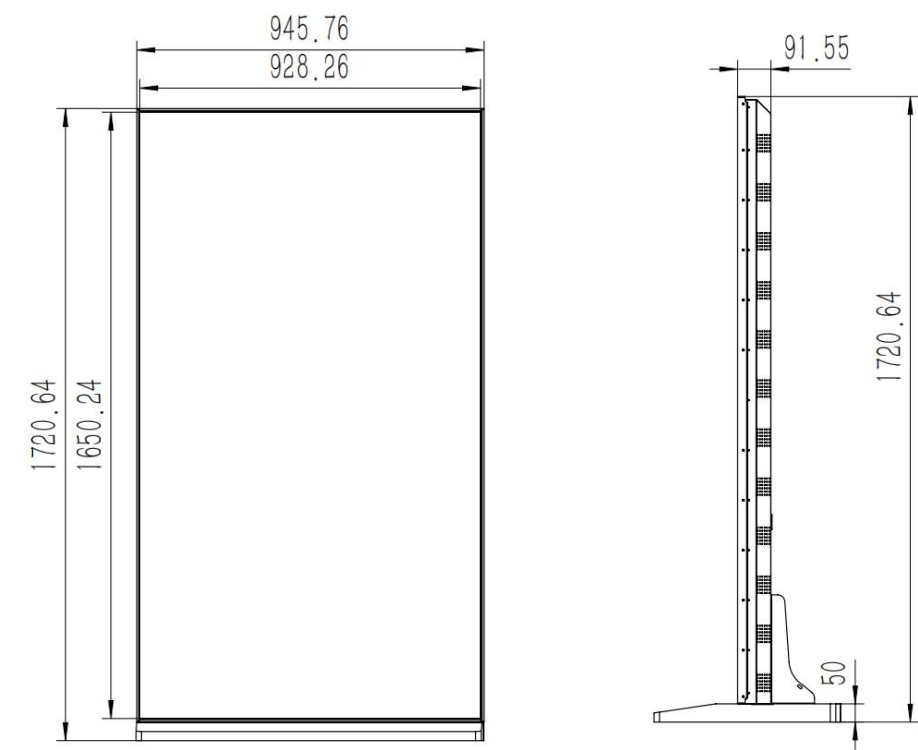
75英寸外观尺寸图
